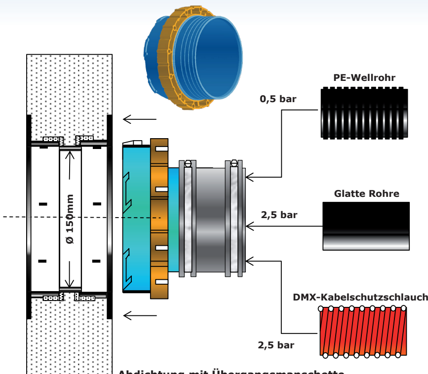
Abdichtung mit Übergangsmanschette für Rohre 50, 63, 75, 110, 125, 140 und 160mm
