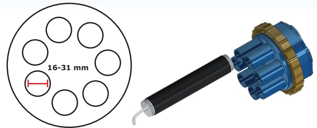
Best.-Nr.: DMS.150.7.33.KS für 7 Kabel von 16-31 mm Inkl. 7x Kaltschrumpfmuffen
