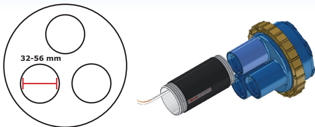
Best.-Nr.: DMS.150.3.58.KS für 3 Kabel von 32-56 mm Inkl. 3x Kaltschrumpfmuffen
