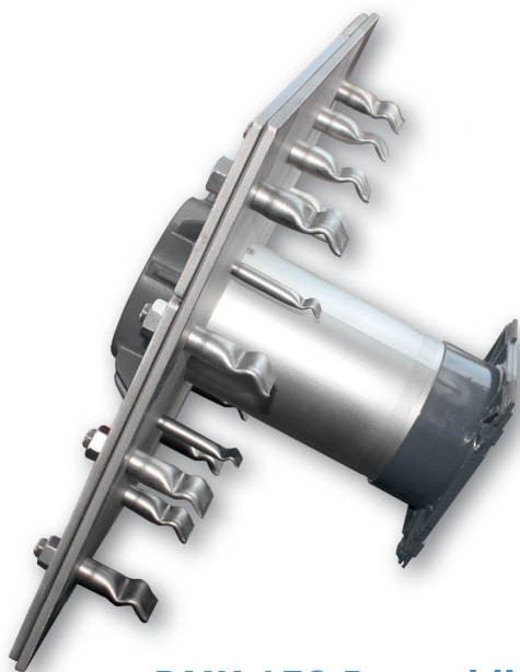
DMK.150 Doppeldichtpackung einseitig mit Fest- Losflansch
