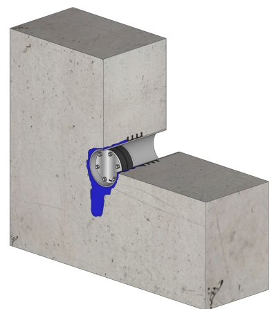
Einbausituation
