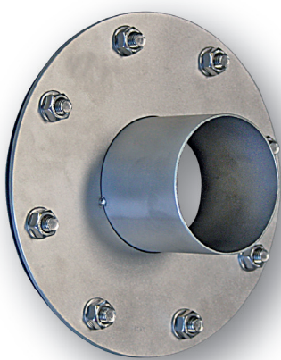
Flanschplatte Edelstahl
