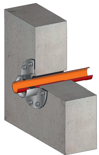
Einbausituation
